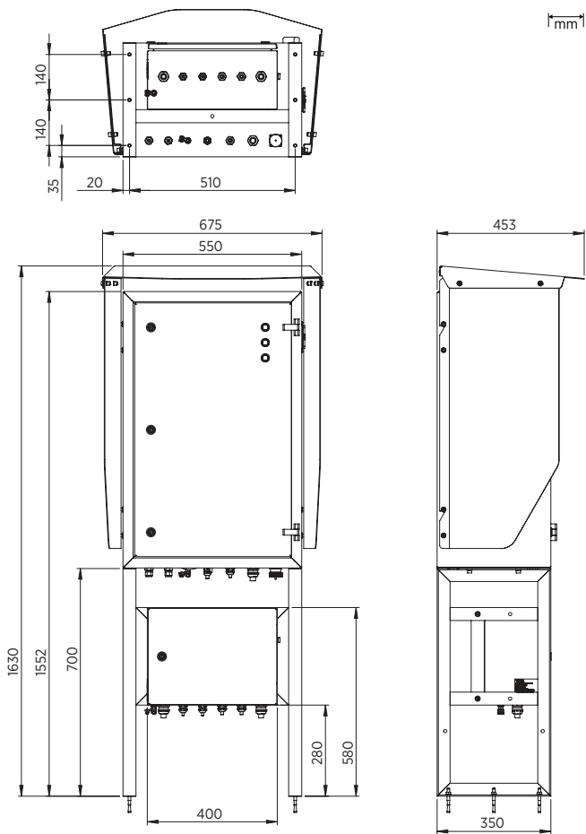
Dimensions
